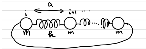
図 2 連成振動
