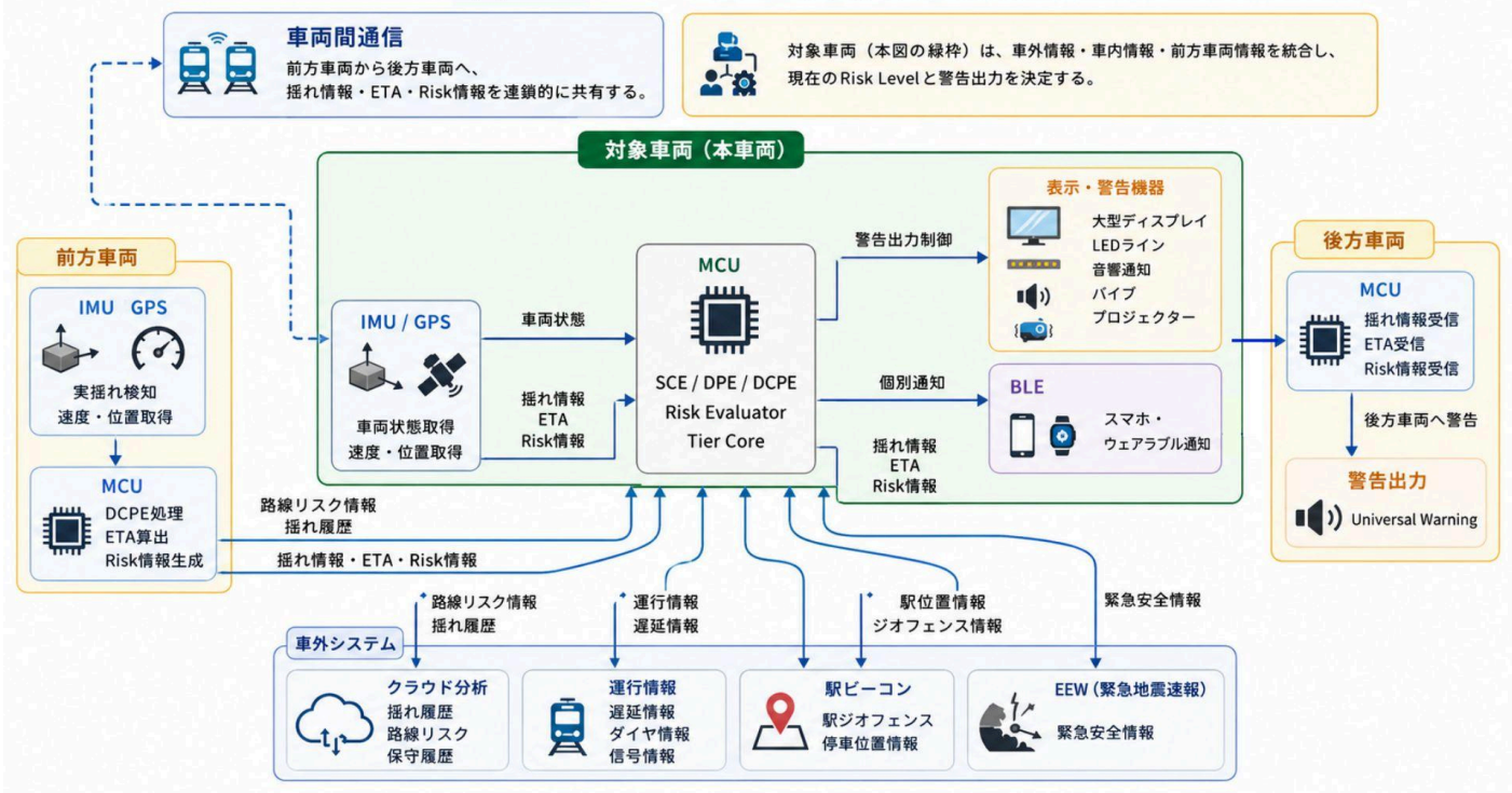
図3-3 URSAS 5.4 車両内外通信系
