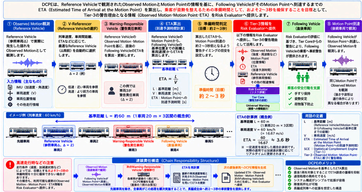
図7-5 DCPE統合制御図
