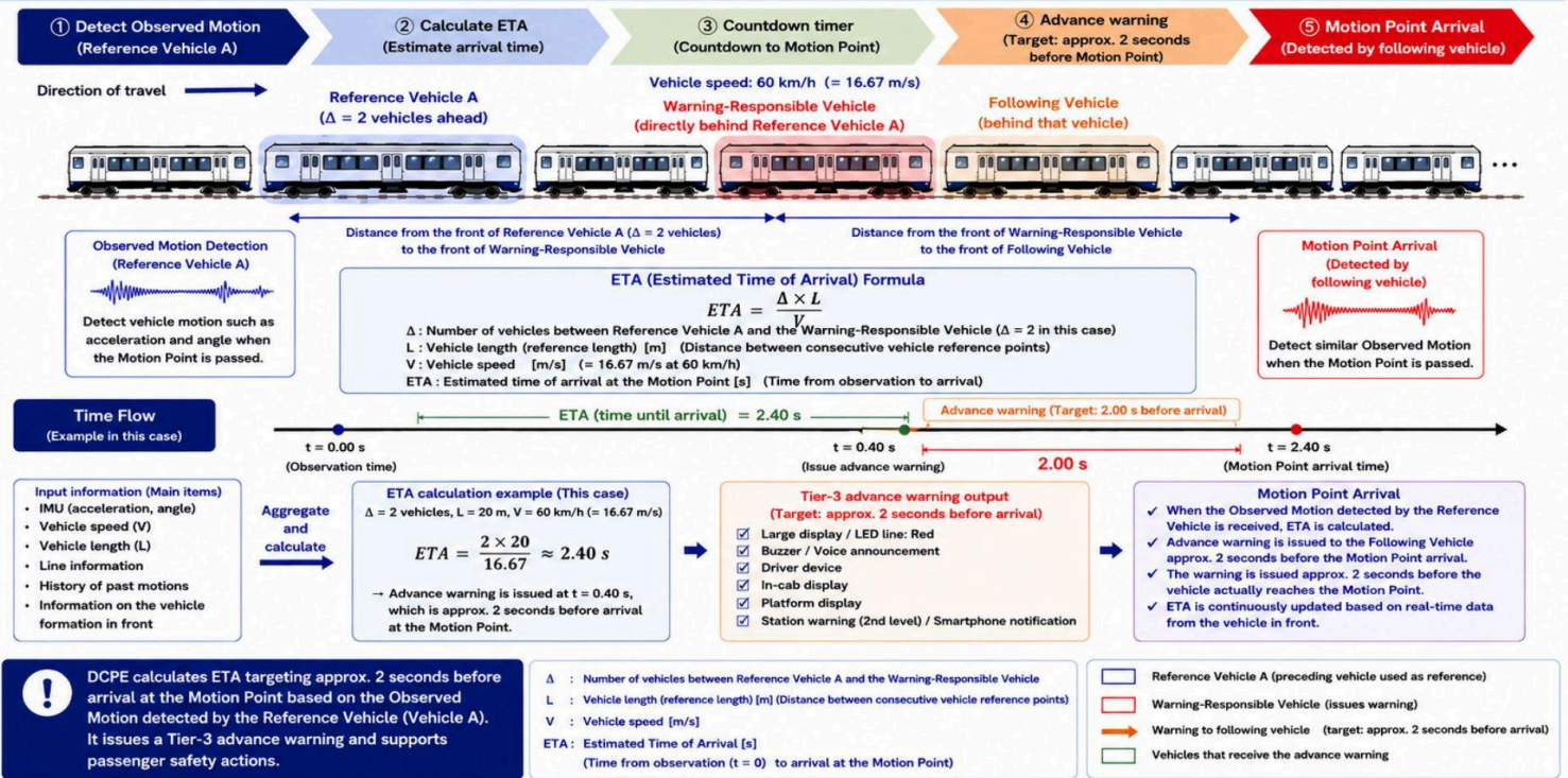
Fig. 7-3 ETA Calculation Model (Revised)
