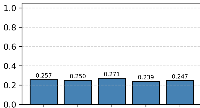
Precision
