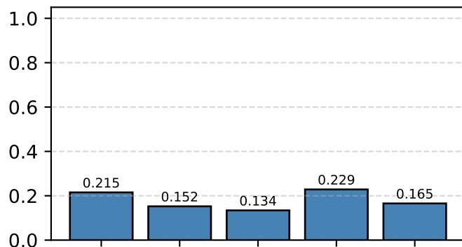
F1
