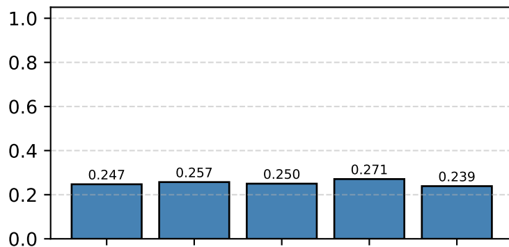
Precision
