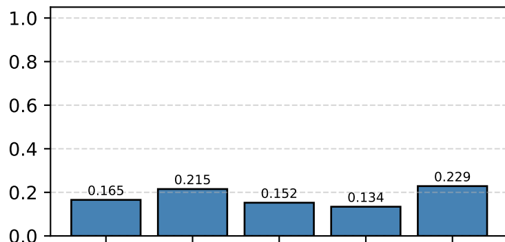
F1
