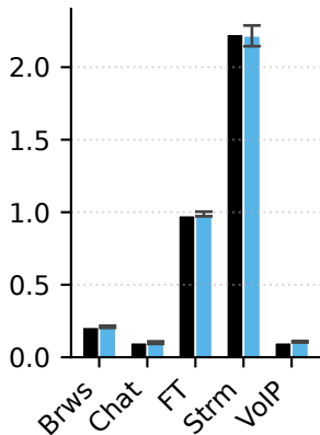
(c) XGBoost VPN shift
