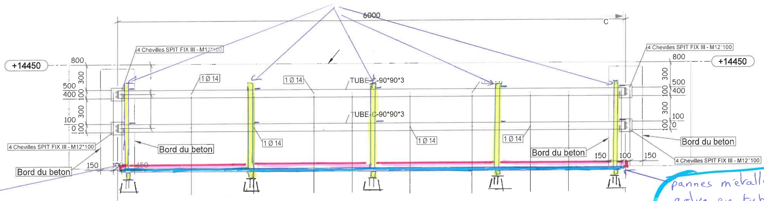
Détail A 1:25
