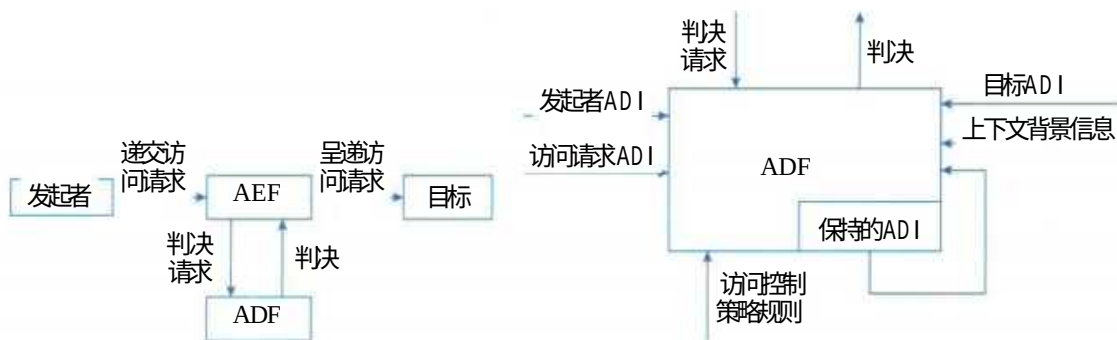
图18-19基本访问控制功能示意图
