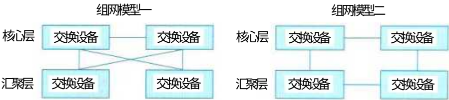
图17-22核心-汇聚层典型组网架构
