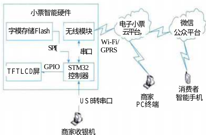
图13-23 电子小票服务系统结构框图
