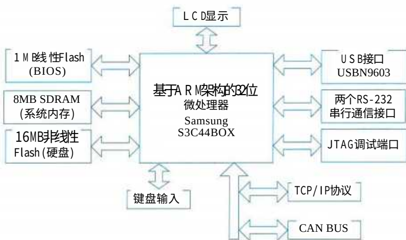
图2-11 基于A R M处理器的嵌入式计算机硬件组成
