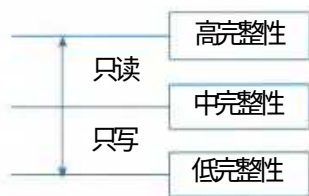
图18-6 Biba模型基本原理
