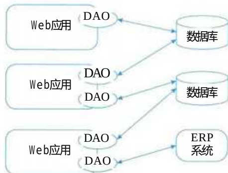
图13-12 DAO 模式
