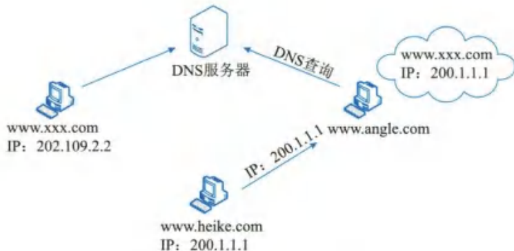
图 4-10 DNS 欺骗
