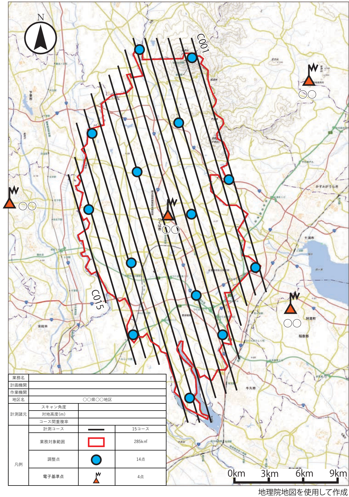
付図記載例（6）「航空レーザ測量等の場合」
