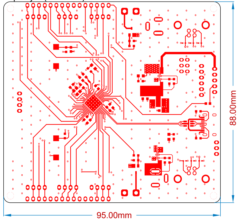
Top Layer (Scale 1:1)
