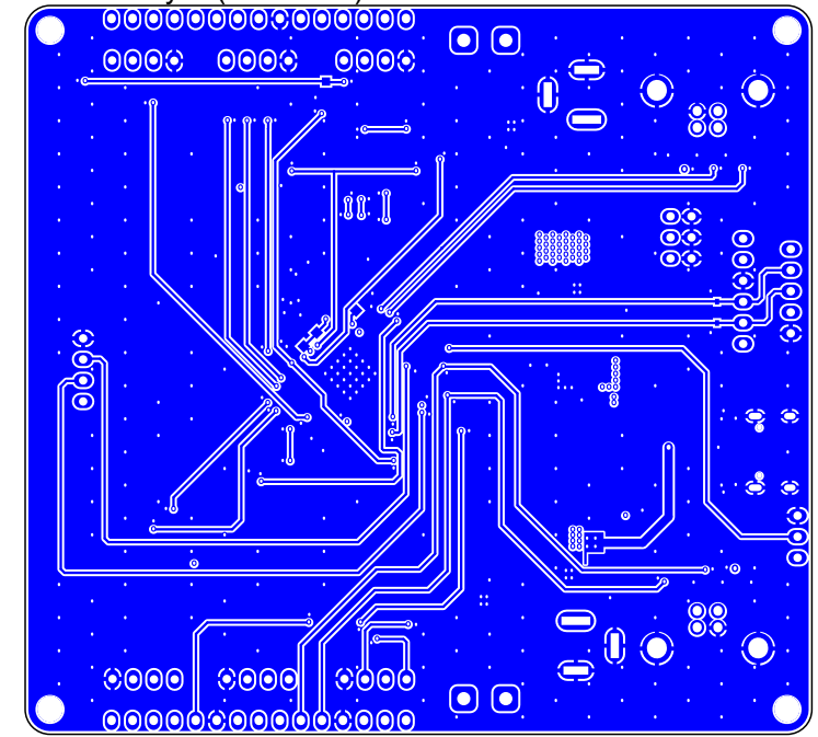
Bottom Layer (Scale 1:1)
