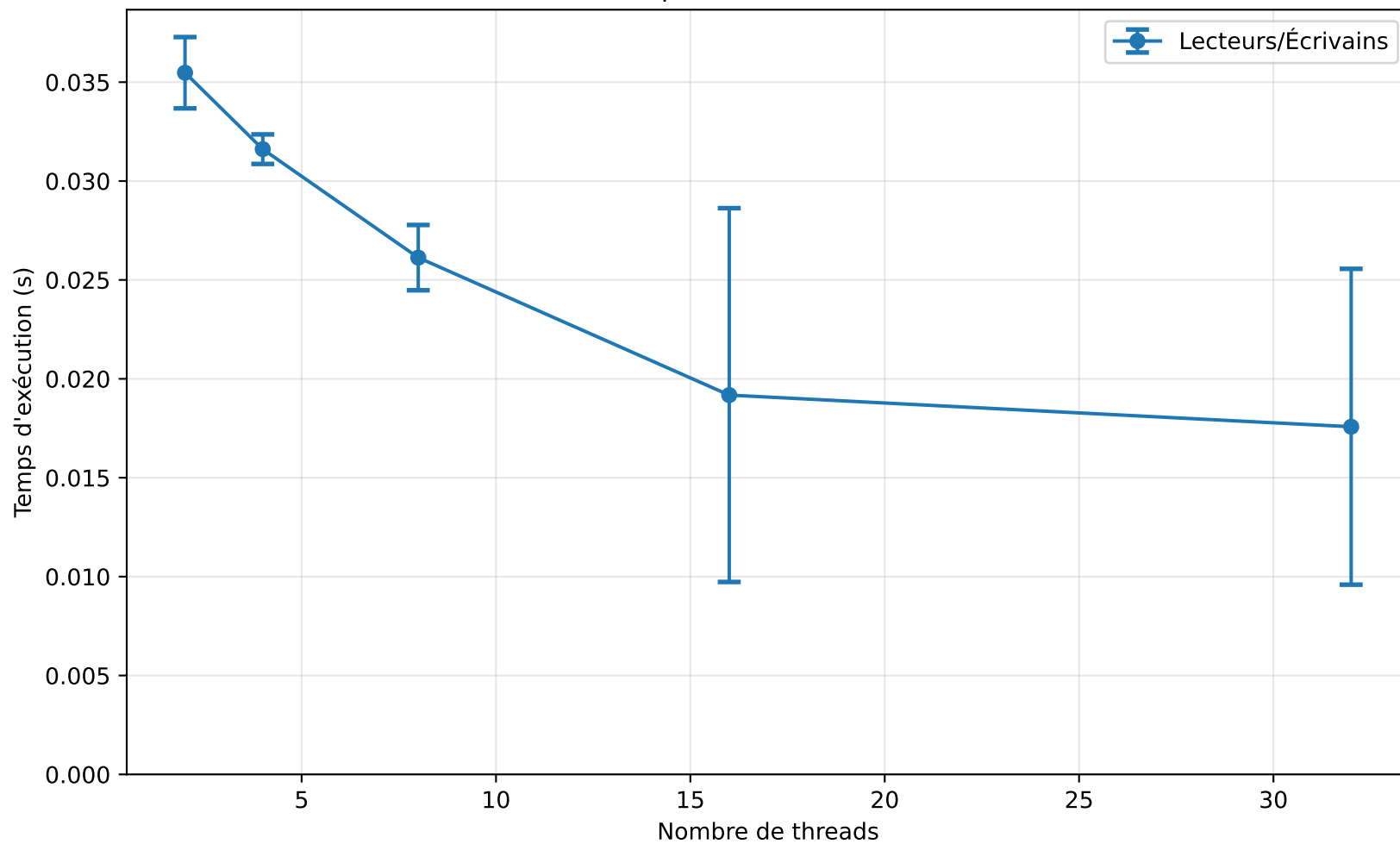
Performance du problème des lecteurs/écrivains
