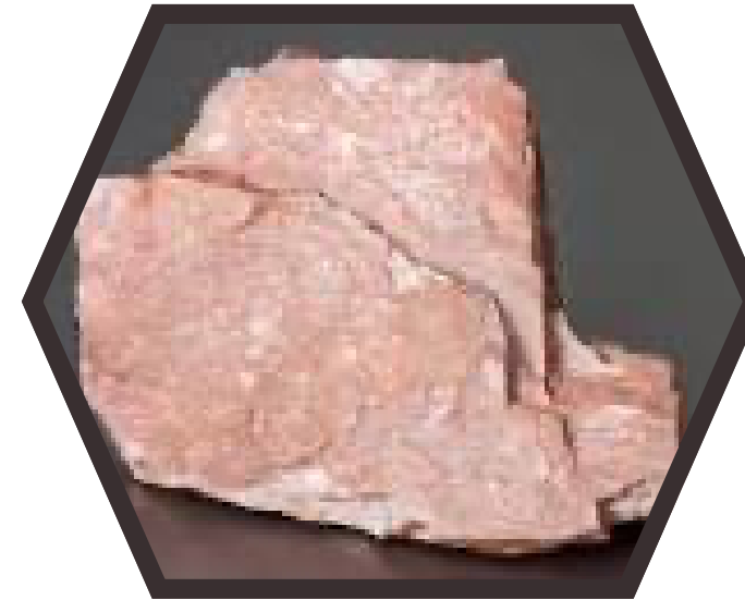
Feldspar
