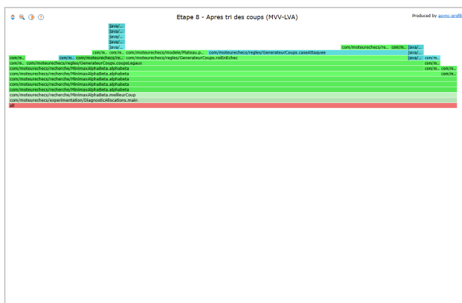
Après tri MVV-LVA (25 319 positions), arbre resserré
