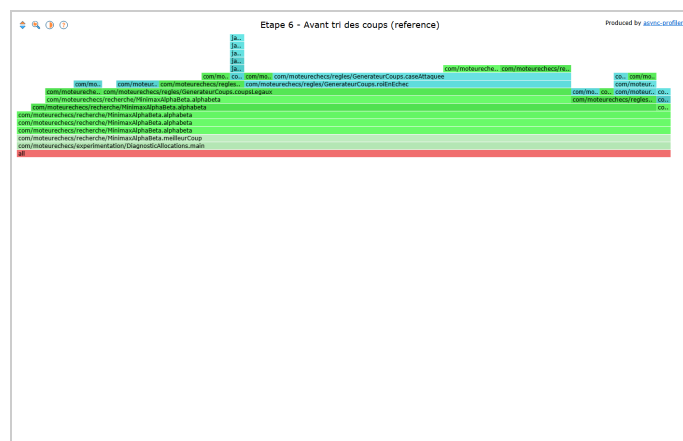
Avant tri des coups (41 554 positions)
