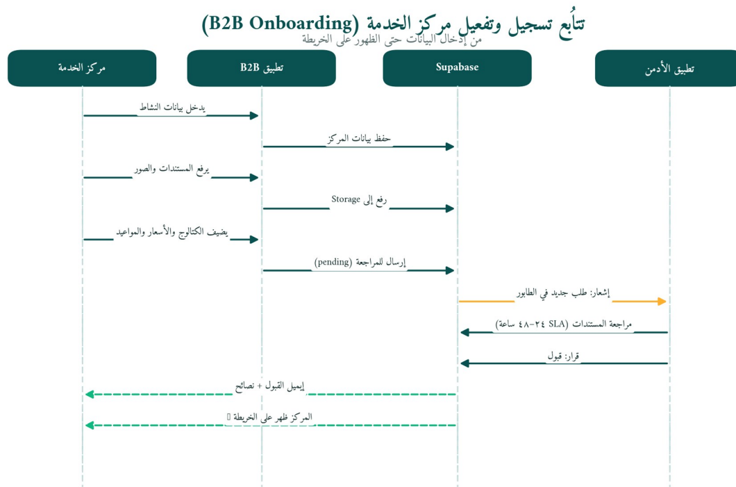
شكل 8: تتابع تسجيل وتفعيل مركز الخدمة (B2B Onboarding).
