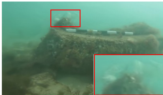
AnySplat
