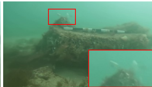
Ours
