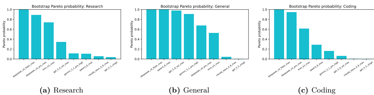
图 5: Bootstrap 抽样下模型进入 Pareto 前沿的概率
