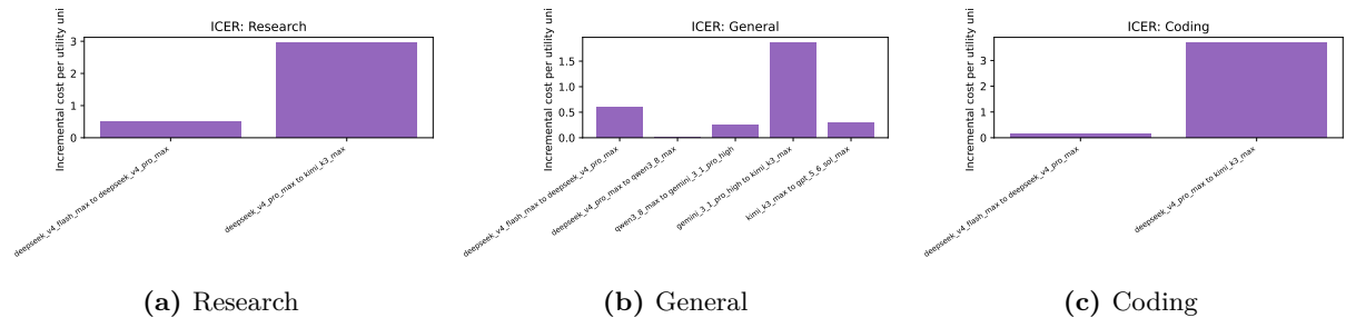
图 3: 三类场景 Pareto 前沿相邻升级的增量成本效益
