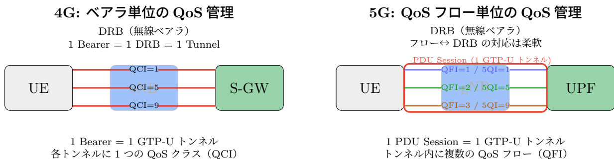
図 2.10: 4G と 5G の QoS モデル比較
