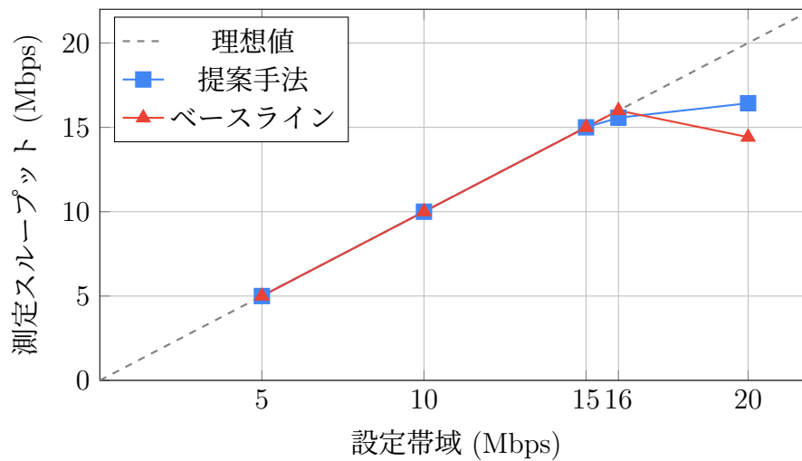
図 7.2: 下り方向 (DL) UDP スループットの比較
