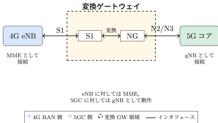
図 4.2: 提案システムの全体構成（S1-N2 変換ゲートウェイ）
