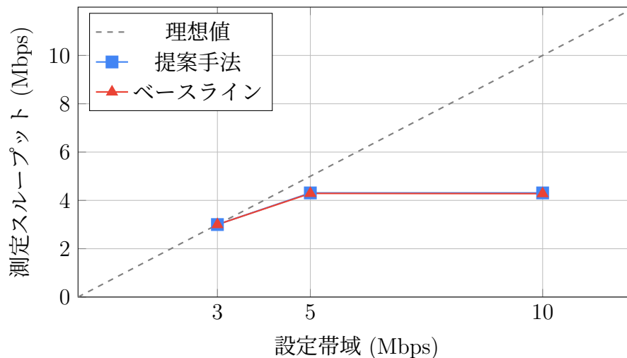
図 7.3: 上り方向 (UL) UDP スループットの比較
