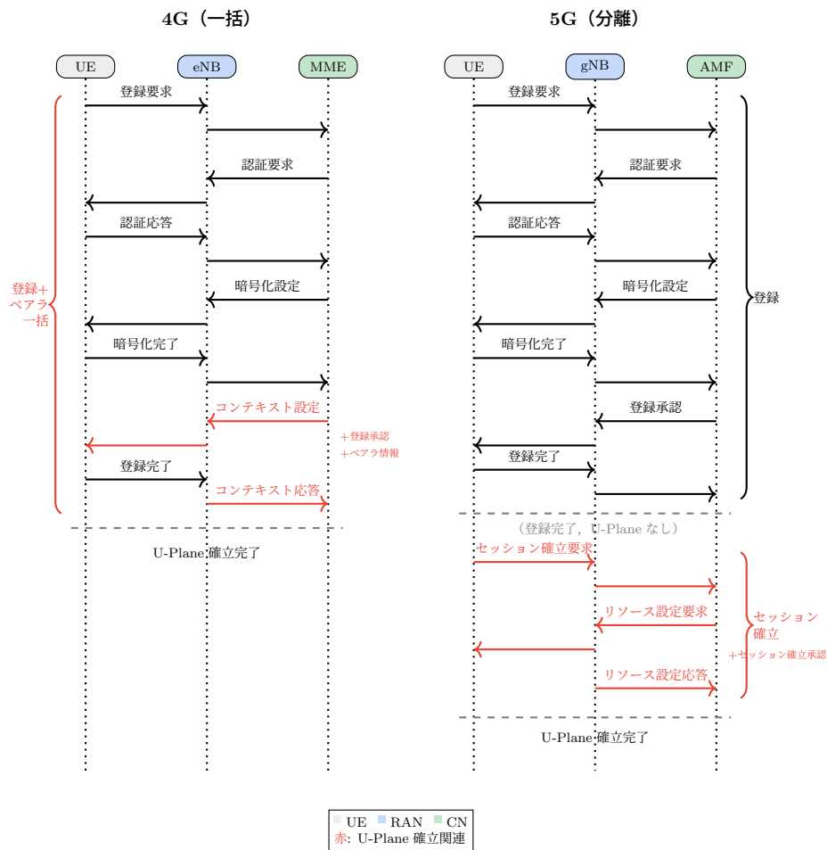
図 2.8: 4G と 5G におけるネットワーク登録から U-Plane 確立までの手順の比較
