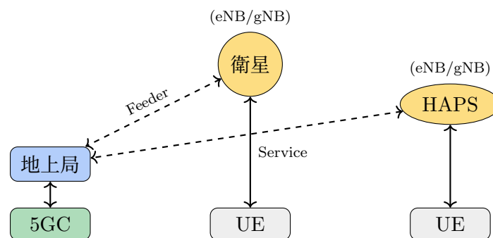
図 7.4: NTN (非地上系ネットワーク) の概念構成
