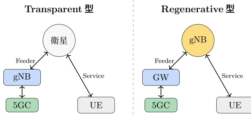
図 7.5: NTN ペイロードアーキテクチャの比較 (TR 38.821[1] に基づく)
