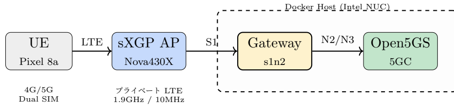
図 5.1: 実験環境構成図. Gateway と Open5GS は同一物理サーバ上の Docker コンテナとして動作する.
