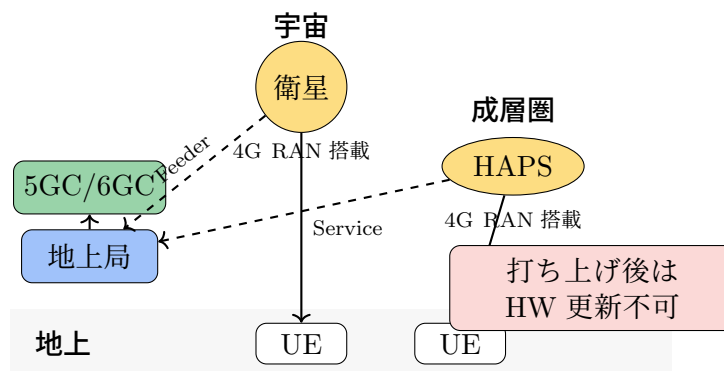
図 2.3: NTN (非地上系ネットワーク) の概念構成
