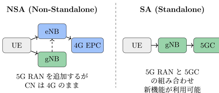
図 2.4: NSA 構成と SA 構成の比較
