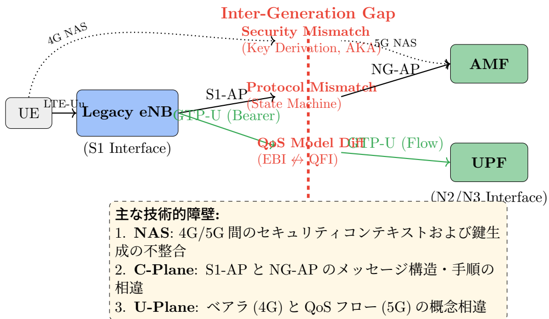
図 2.5: レガシー RAN と 5GC 間の技術的ギャップ
