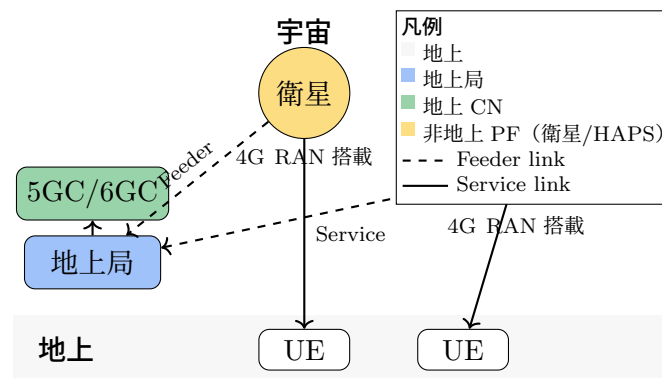
図 7.3: NTN（非地上系ネットワーク）の概念構成
