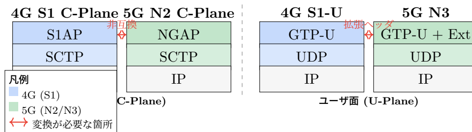
図 2.6: 4G (S1) と 5G (N2/N3) のプロトコルスタック比較
