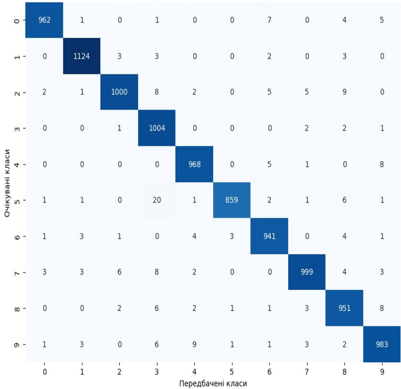
Матриця плутанини (Confusion Matrix) для 10 класів
