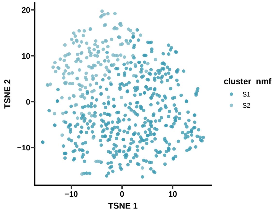
TSNE
