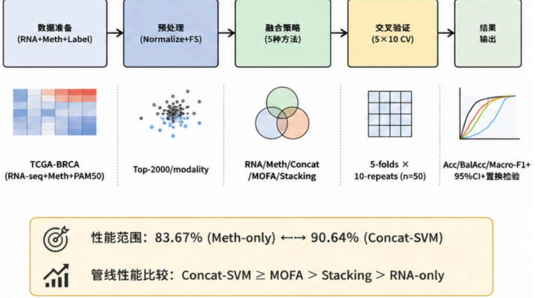
图 9: 融合方法实验管道总览。展示从数据读取、样本对齐、训练-测试划分到各融合分支训练的完整流程。所有可学习步骤（特征筛选、标准化、MOFA 拟合、Stacking 元特征构造）均限定在训练折内完成，测试折仅用于独立推断，严格遵循防泄露原则。
