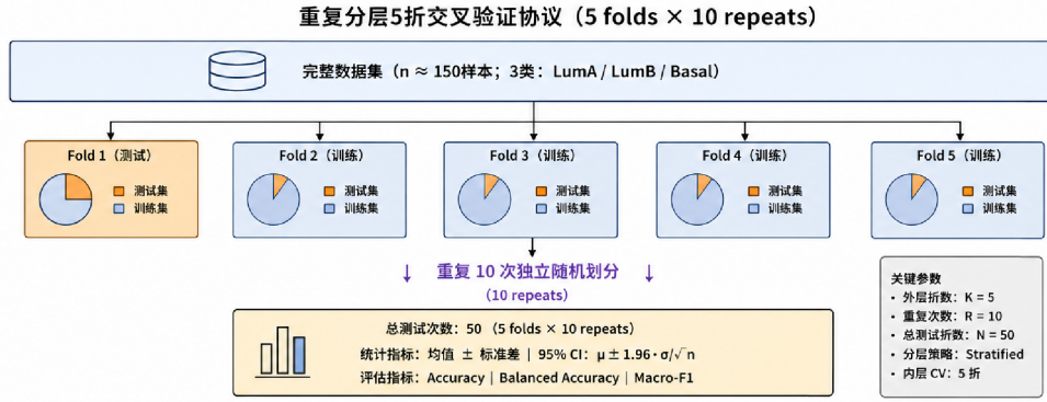
图 10: 重复分层交叉验证协议示意图。主实验采用 5 折 10 次重复, n = 50 测试折, 分层策略确保每个折内各类别比例与总体分布一致。外层 Loop 控制数据划分, 内层 Loop 在训练折内完成特征筛选与模型训练, 测试折仅用于独立推断。
