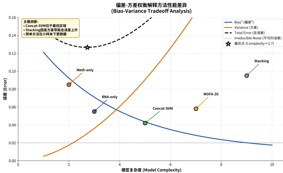
图 18: 偏差-方差权衡分析。在小样本高维场景，样本约 150，特征远多于样本，复杂模型 Stacking 虽然偏差较低，但方差显著增大，导致总体泛化误差上升。简单模型 Concat-SVM 通过限制模型复杂度，实现了更优的偏差-方差权衡。
