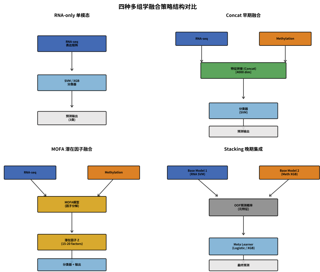
图 5: 四种融合策略（RNA-only、Concat、MOFA、Stacking）的架构对比。自上而下展示各方法的输入模态、融合机制与分类器结构。RNA-only 仅使用转录组数据作为单模态基线；Concat 将 RNA 与甲基化特征直接拼接；MOFA 通过潜在因子压缩冗余；Stacking 在分支级决策基础上进行元融合。
