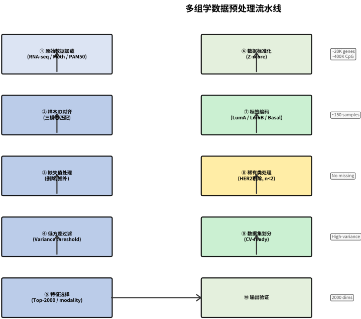
图 3: 数据预处理管道流程。涵盖 RNA-seq 对数变换与甲基化缺失值处理、均值过滤、方差排序及标准化等关键步骤。预处理顺序严格遵循防泄露原则，所有参数估计均在训练折内完成。
