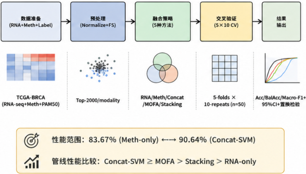
图 9: 融合方法实验管道总览。展示从数据读取、样本对齐、训练-测试划分到各融合分支训练的完整流程。所有可学习步骤（特征筛选、标准化、MOFA 拟合、Stacking 元特征构造）均限定在训练折内完成，测试折仅用于独立推断，严格遵循防泄露原则。
