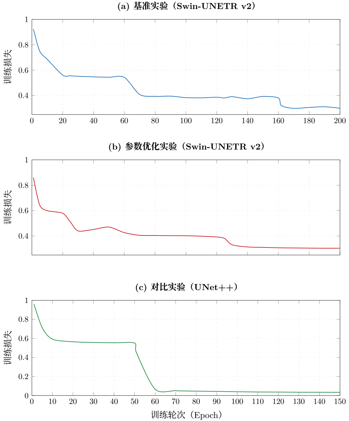
图 4. 三组独立实验的训练损失曲线。(a)(b) Swin-UNETR v2 呈现两阶段收敛特征，损失从 \sim 0.9 降至 \sim 0.30 ；(c) UNet++ 在第 50-60 轮间出现急剧下降（从 0.55 降至 0.07），最终收敛至 0.034，远低于 Swin-UNETR v2。
