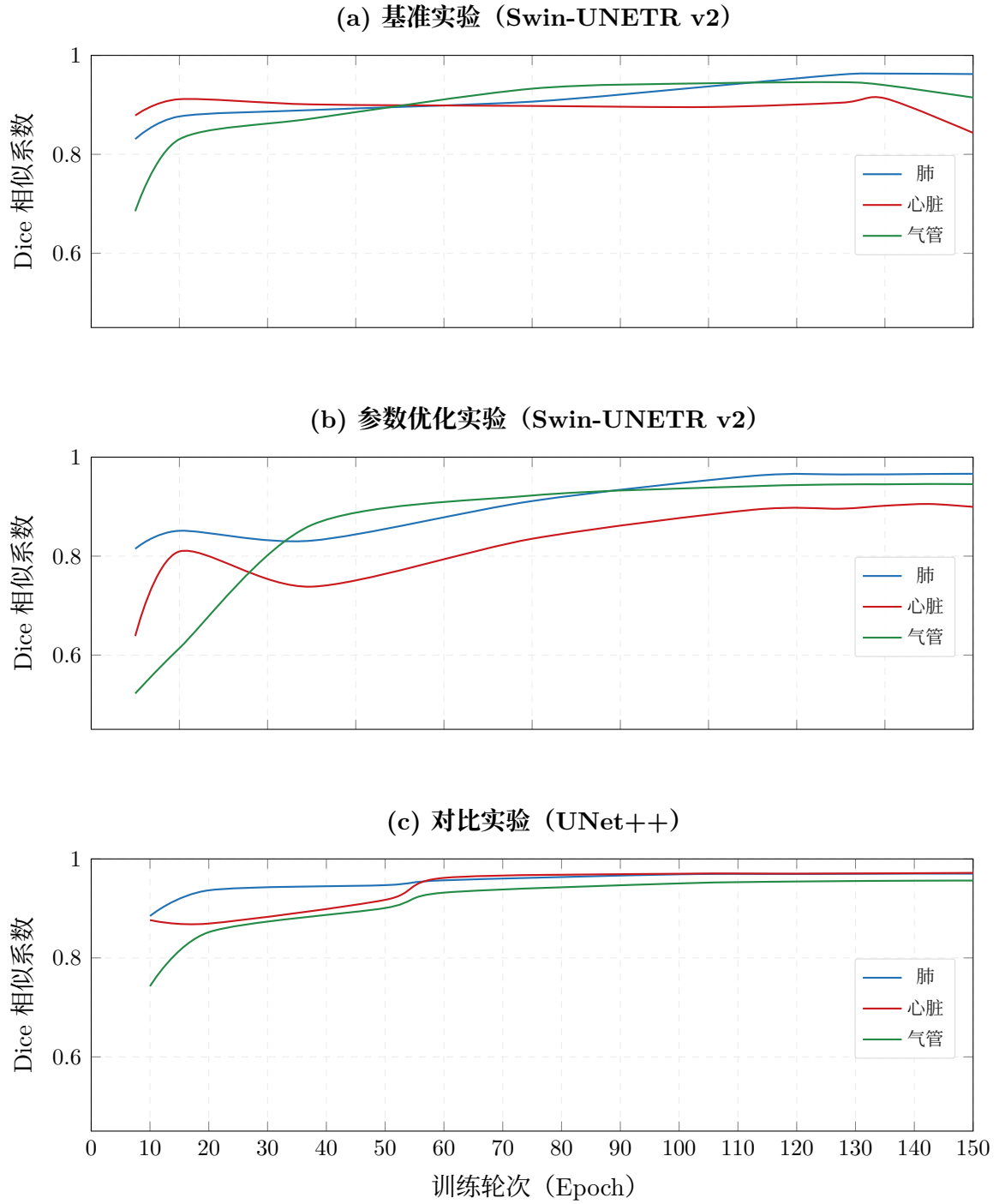
图 5. 三组独立实验各器官 Dice 系数变化趋势。(a)(b) Swin-UNETR v2 中肺收敛最快，心脏与气管后期波动明显；(c) UNet++ 中三类器官均在第 60 轮后快速收敛至 0.95 以上，心脏 DSC 甚至超过肺，展现出优异的分割性能。
