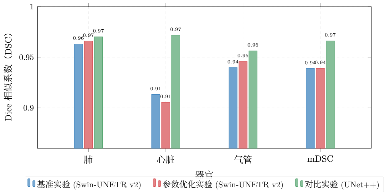
图 6. 三组独立实验最佳模型各器官 DSC 对比。UNet++ 在所有器官上均优于 Swin-UNETR v2，心脏分割提升最为显著（+5.86pp）。
