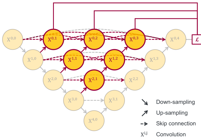
图 3. UNet++ 架构示意图。图中 X_{i,j} 表示第 i 层第 j 个卷积块。虚线表示跳跃连接, 实线表示降采样/上采样路径。UNet++ 通过在编码器与解码器之间引入密集卷积块 (橙色节点), 逐步缩小语义差距。
