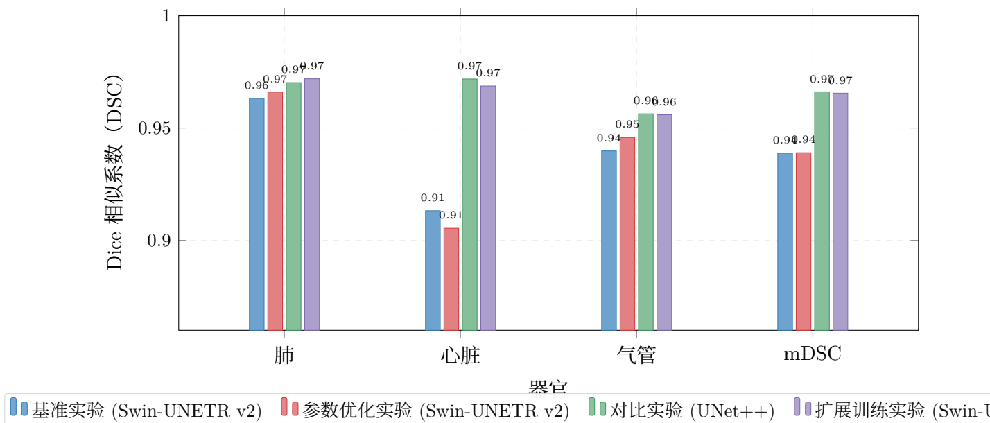
图 6. 四组独立实验最佳模型各器官 DSC 对比。UNet++ 取得最高 mDSC (0.9661)，扩展训练的 Swin-UNETR v2 紧随其后 (0.9655)，两者差距仅 0.0006。扩展训练实验在肺部 DSC 上取得最高值 (0.9719)。
