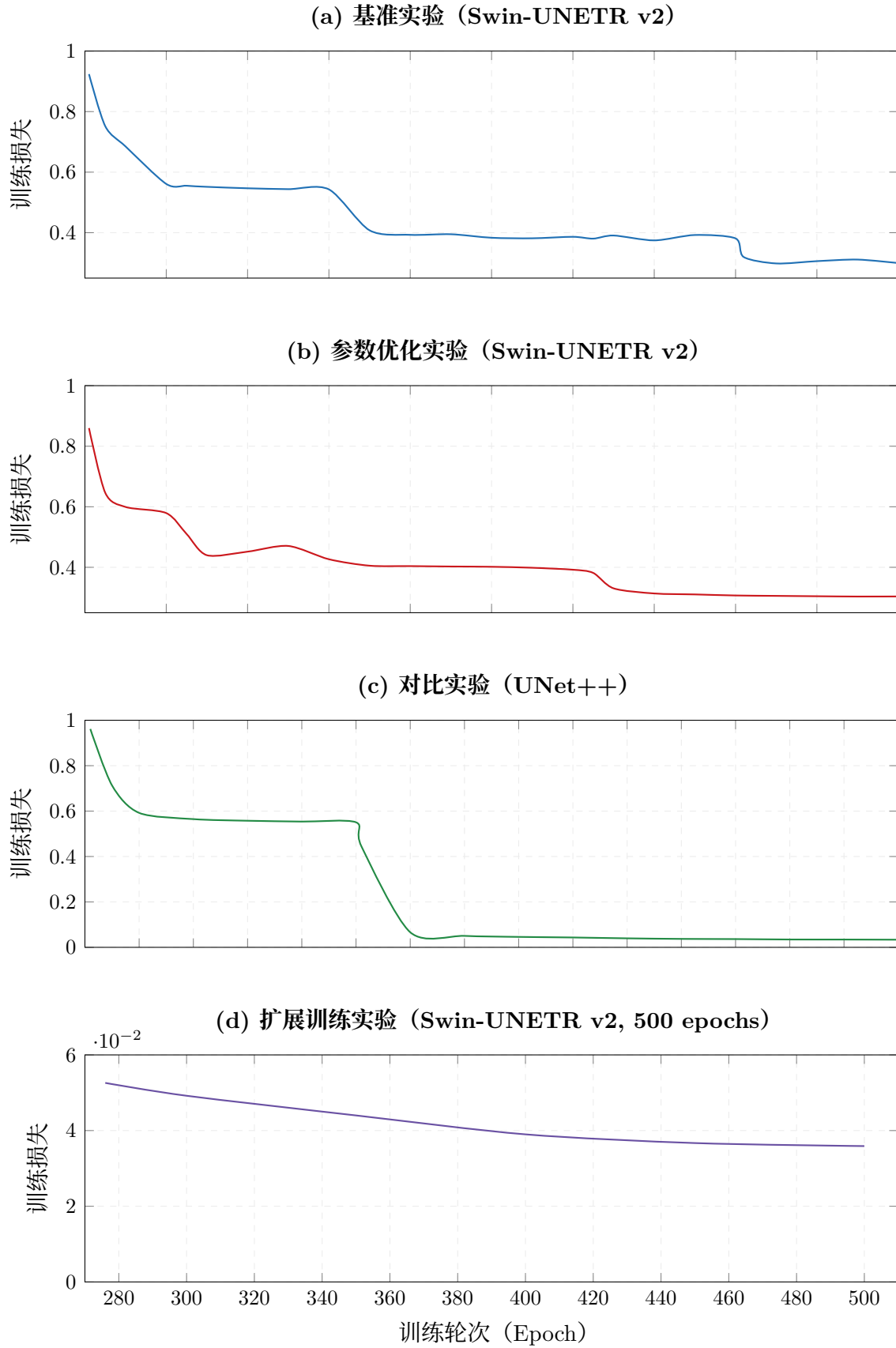
图 4. 四组独立实验的训练损失曲线。(a)(b) Swin-UNETR v2 呈现两阶段收敛特征，损失从 \sim 0.9 降至 \sim 0.30 ；(c) UNet++ 在第 50-60 轮间出现急剧下降（从 0.55 降至 0.07），最终收敛至 0.034；(d) 扩展训练实验从第 276 轮继续训练，损失从 0.053 缓慢收敛至 0.036，表明模型在更长训练周期下持续优化。
