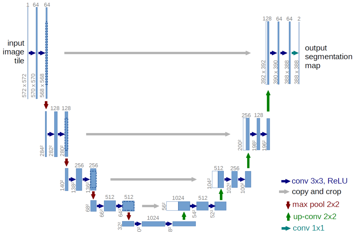
图 1. U-Net 架构示意图。编码器通过最大池化逐步降低空间分辨率并增加特征通道数；解码器通过转置卷积恢复空间分辨率；跳跃连接将编码器特征与解码器特征拼接，保留细节信息。
