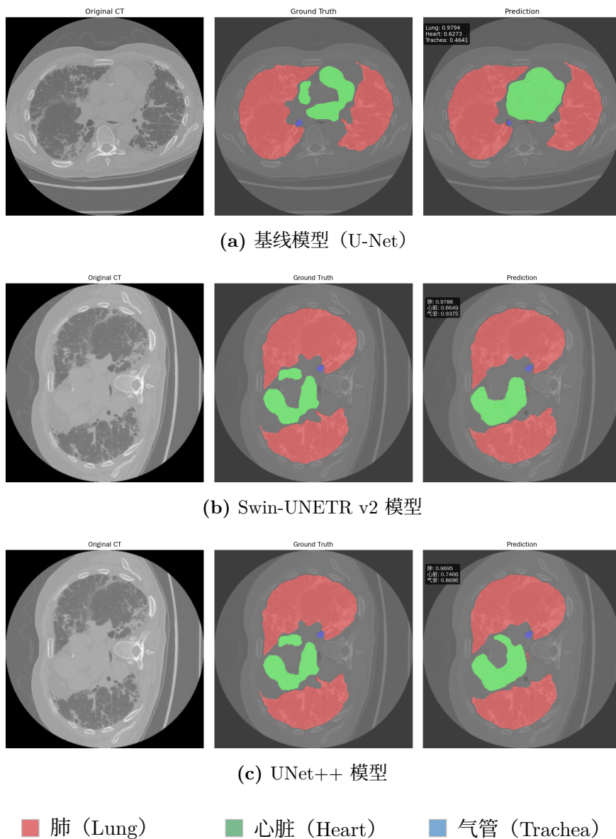
图 7. 三种模型的分割可视化结果对比。从上到下依次为: (a) 基线模型 (U-Net), (b) Swin-UNETR v2 模型, (c) UNet++ 模型。每个子图包含原始 CT 图像、真实标注和模型预测三列。红色表示肺部区域, 绿色表示心脏区域, 蓝色表示气管区域。
