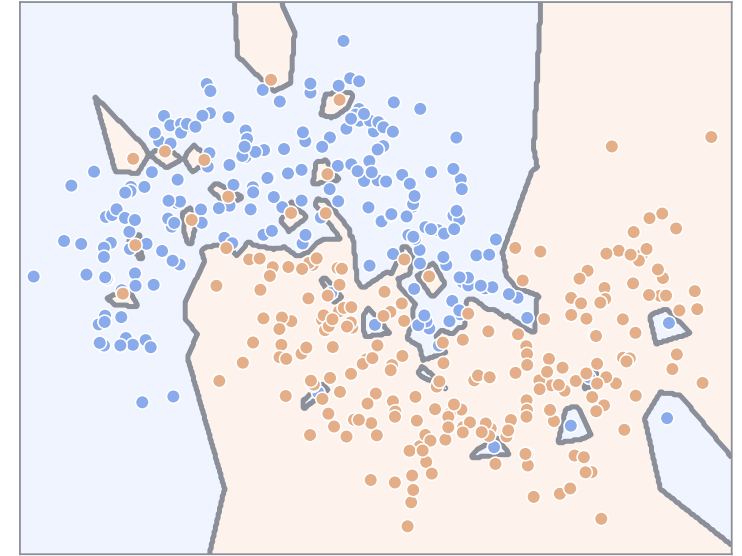
Переобучение
