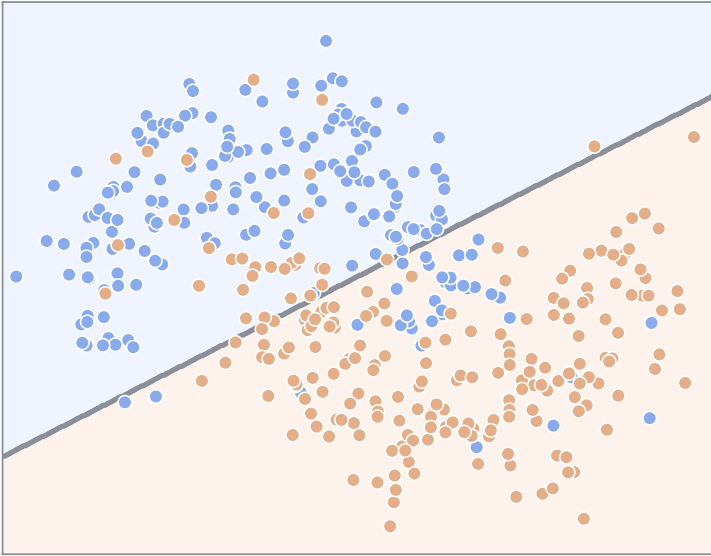
Недообучение
