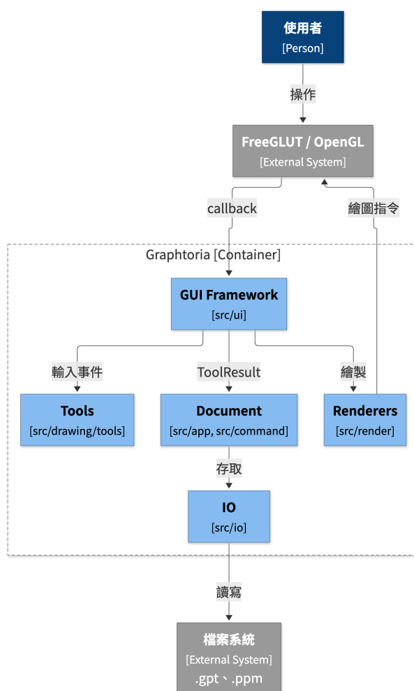
Figure 18: Graphtoria 的 C4 Component 圖
