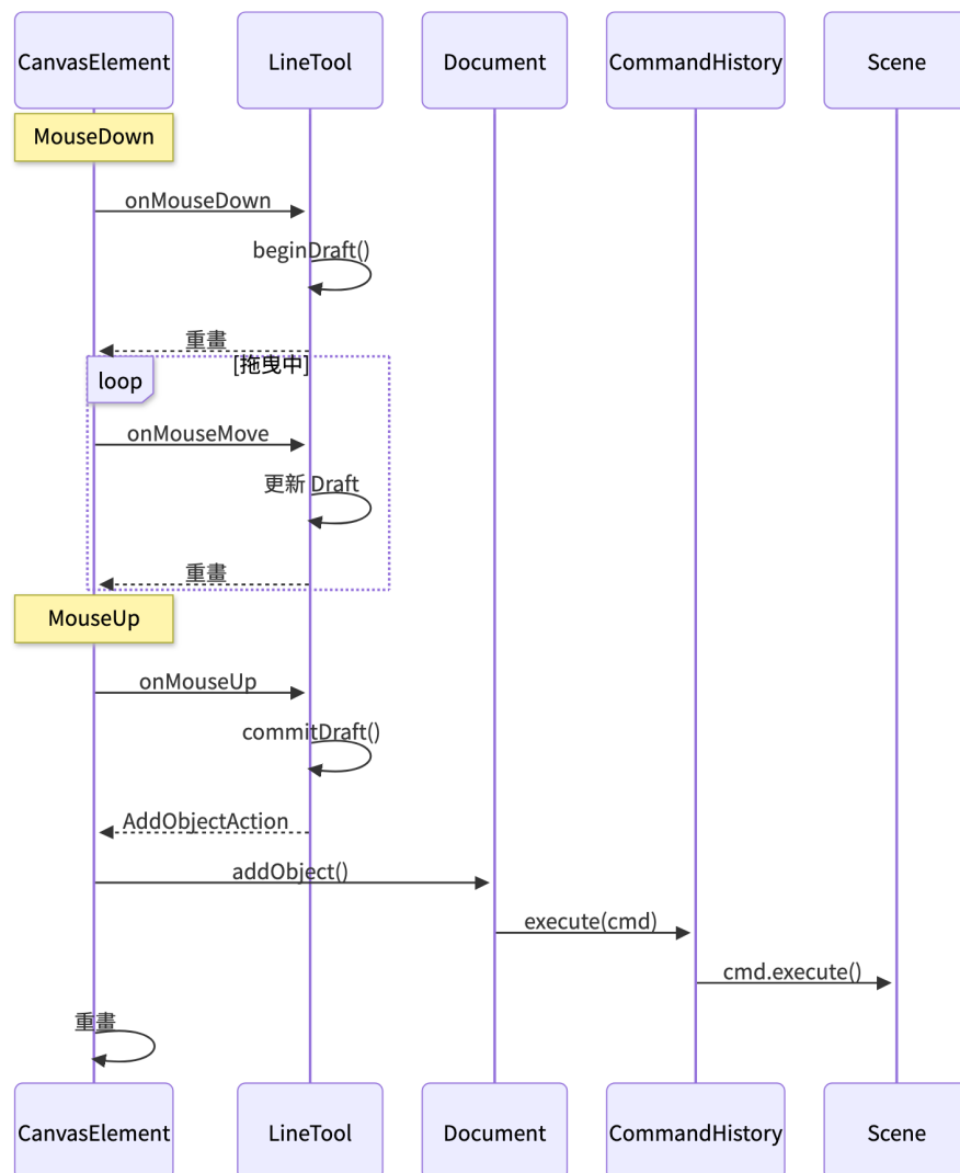
Figure 22: 以 Line 工具繪製一條直線的循序圖
