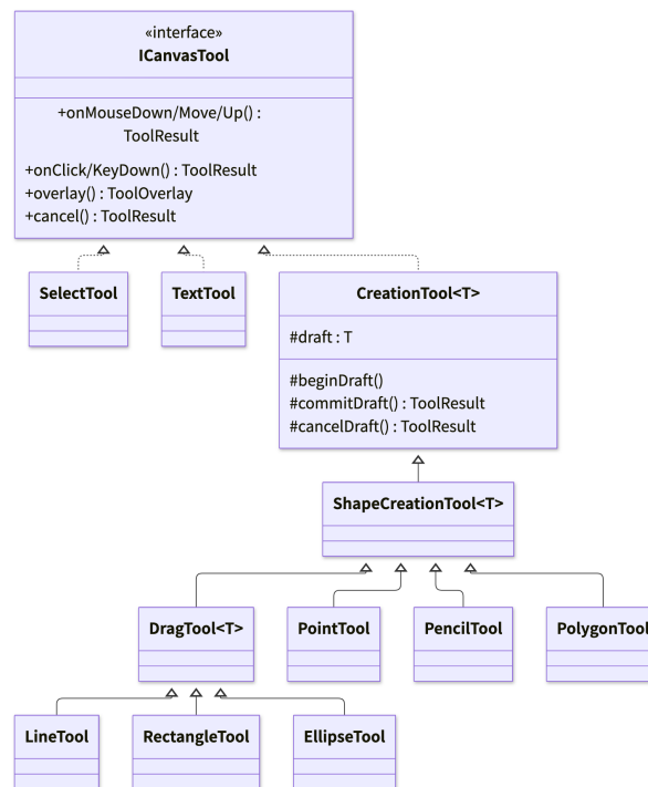
Figure 21: 繪圖工具的類別圖
