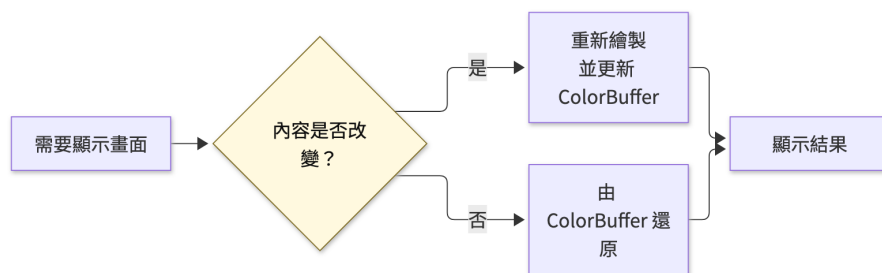
Figure 11: display callback 依內容是否改變，選擇重新 render 或由 ColorBuffer 還原
