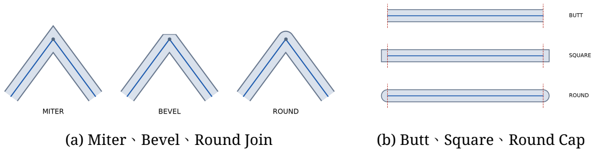
Figure 6: 程式支援的 Line Join 與 Line Cap
