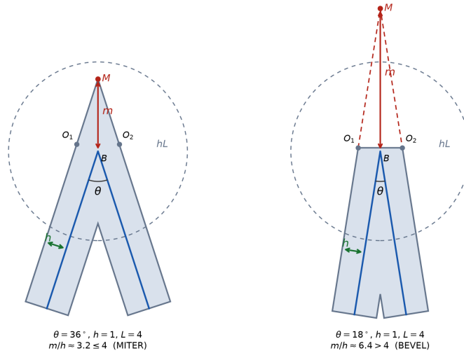
Figure 7: Miter 長度在限制內與超過限制時的處理
