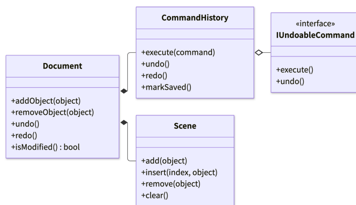
Figure 19: Document 與 Command 的類別圖
