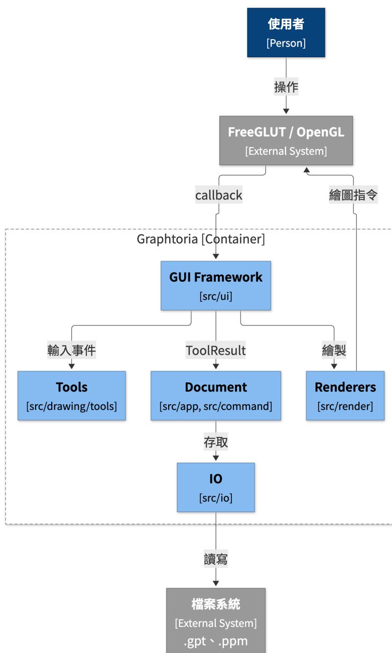
Figure 18: Graphtoria 的 C4 Component 圖
