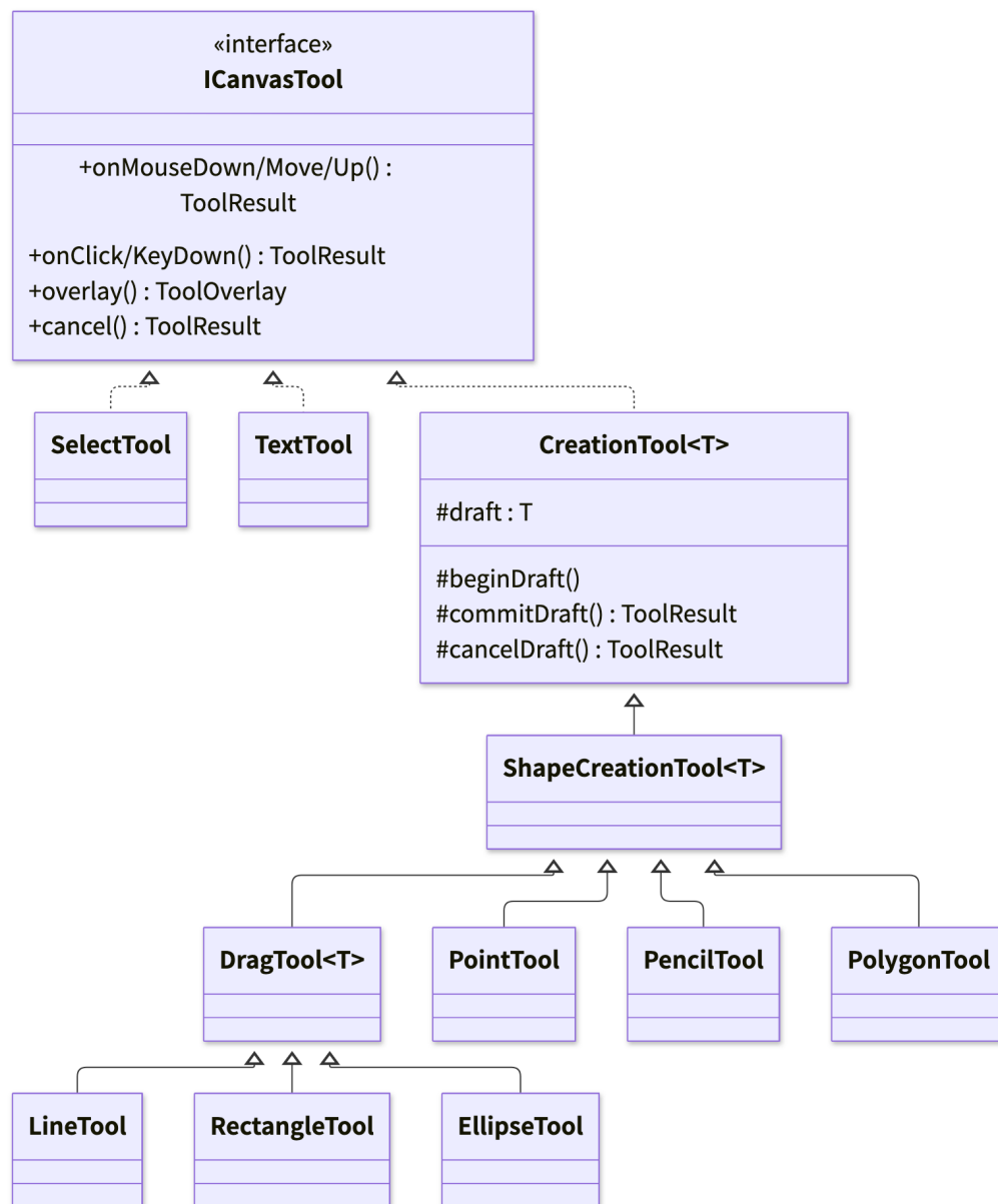
Figure 21: 繪圖工具的類別圖
