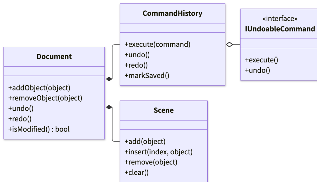
Figure 19: Document 與 Command 的類別圖
