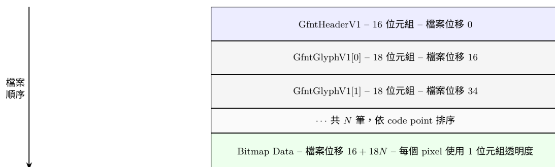
Figure 17: GFNT v1 二進位檔案配置
