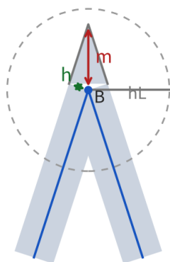
Figure 7: Miter limit 的實際轉角案例；灰底表示筆畫寬度，藍線為中心線
