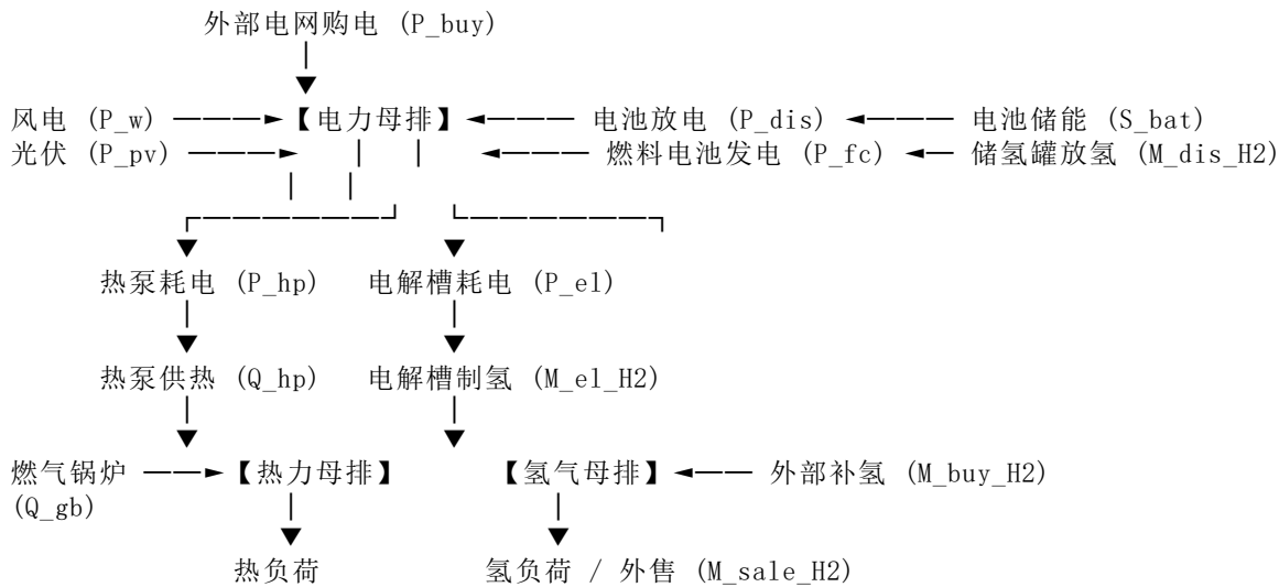
图 1：电-热-氢-储综合能源系统耦合网络拓扑
