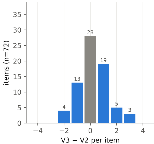
Gemma 4 31B-IT
