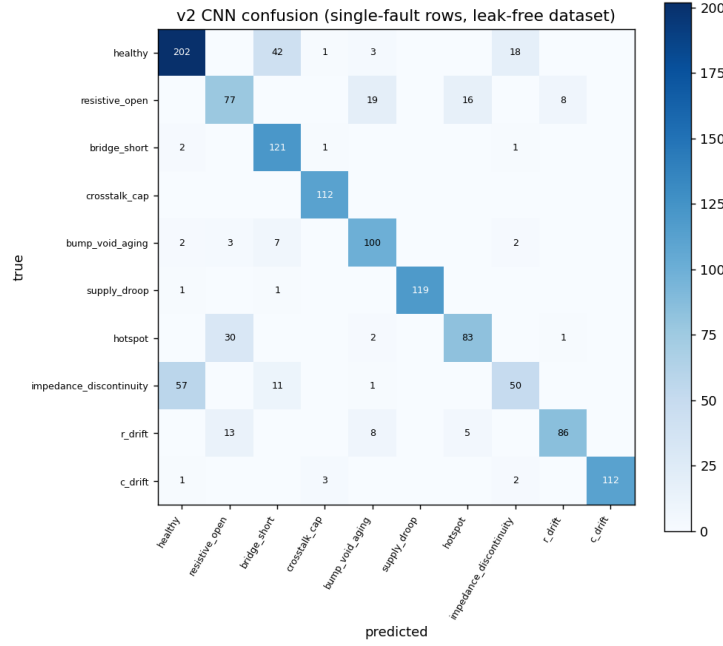
图 3: CNN 的混淆矩阵（单故障子集）。残余混淆对应物理上的机制简并：近标称阻抗台阶 \approx 健康、热点 \approx 局部串阻、两类凸点/导线串阻故障在重叠幅度区间不可分。
