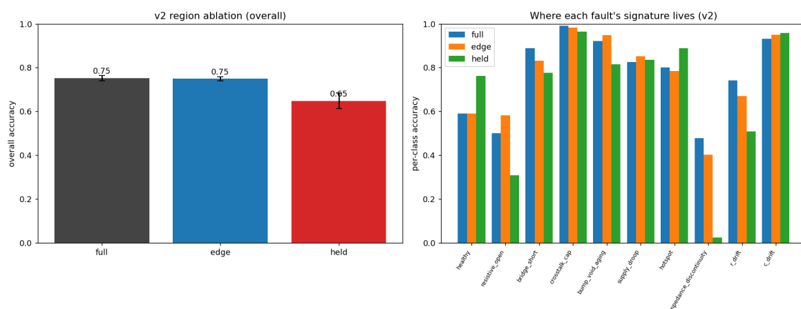
图 5：区域消融。左：总体准确率（3 次重初始化，误差棒为标准差）；右：逐类准确率—— impedance_discontinuity 在仅平台区下降至 0.03，健康类反而在平台区更高。
