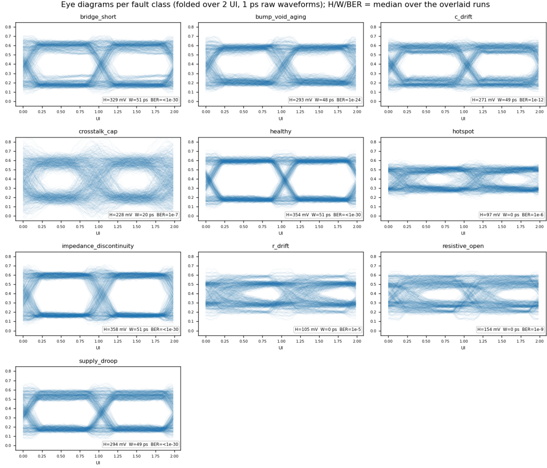
图 2: 每类故障的接收端眼图（折叠 2 UI，由 1 ps 分辨率原始波形绘制，而非机器学习输入用的 8 样 / UI 重采样版本——后者每个跳变沿仅约 2.4 个采样点，画出的眼会呈折线状）。每幅子图右下角标注所叠加各次运行的眼高 H （最坏情形垂直开口 \min(\text{高电平}) - \max(\text{低电平}) ）、眼宽 W （UI 减峰峰抖动）与按 Q 因子高斯外推的 BER 的中位数； \text{BER} < 10^{-30} 表示外推值低于可显示范围（见第 3.1 节关于 BER 饱和性的讨论）。阻抗不连续属反射域故障，在幅度域几乎不可见，对应后文区域消融中其“仅平台区准确率 0.03”的结果。
