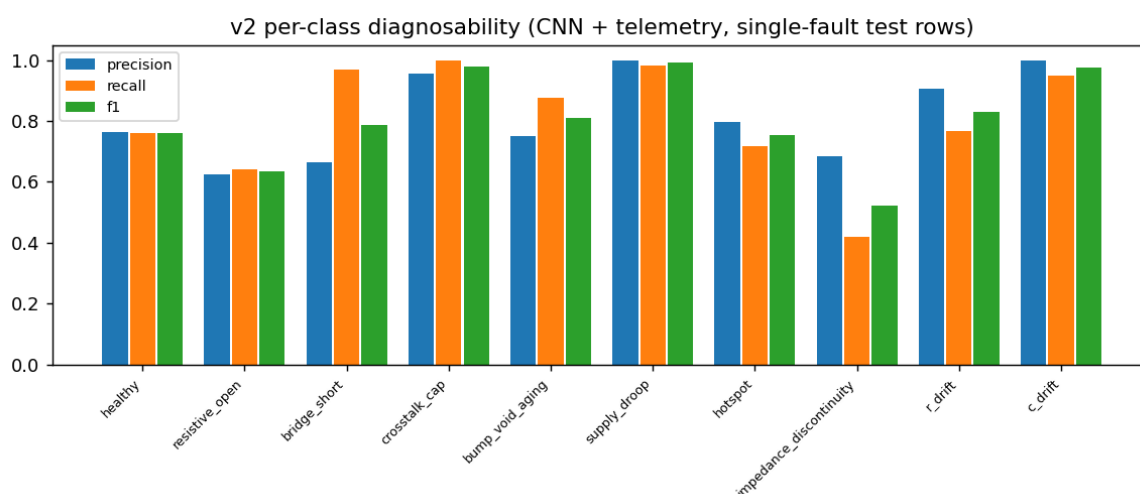
图 6: 逐类精确率/召回率/F1 (CNN+ 遥测, 单故障测试行)。三档可分性: 供电跌落/串扰/ c_drift 为最高档; 衰减族内部互混; impedance_discontinuity 召回降至 0.420 (57 例漏为 healthy )。
