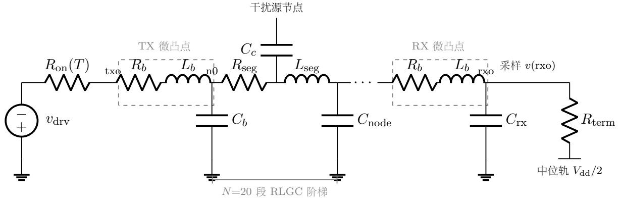
图 1: 受害信号道的 ngspice 等效电路 (单端)。温度相关驱动 R_{on}(T) 启动 PWL 摆; 信号经 TX 微凸点 ( R_b + L_b + C_b )、 N=20 段 RLGC 阶梯 (逐节点对地电容 C_{node} , 并经 C_c 与相邻干扰源耦合)、RX 微凸点, 到达接收节点 ( C_{rx} + 终端 R_{term} 接中位电平 V_{dd}/2 )。故障注入即在指定段位修改 R_{seg} 、 L_{seg} 、 C_{node} 、 C_c 或驱动摆幅 (见表 1)。
