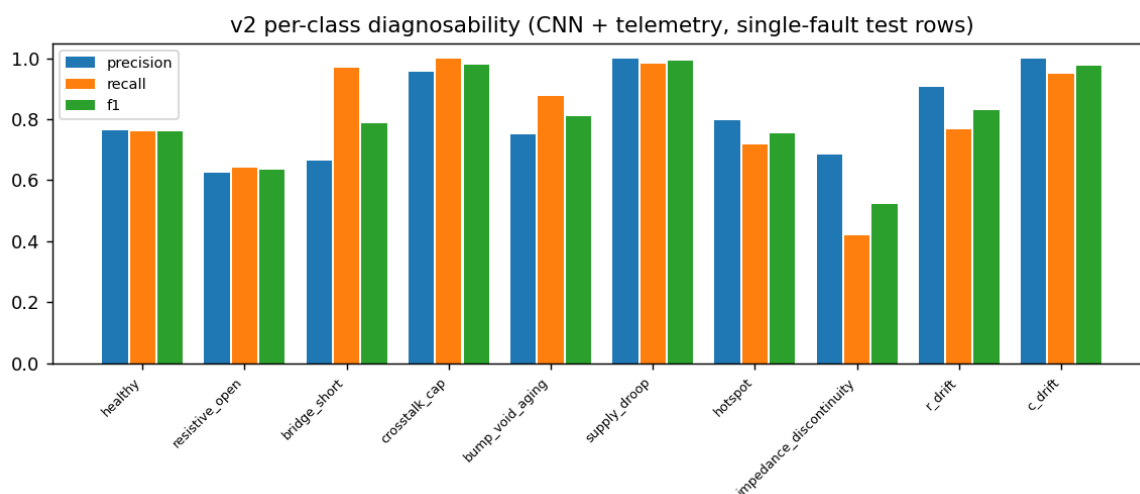
图 6: 逐类 precision / recall / F1 (CNN+ 遥测, 单故障测试行)。三档可分性: droop/串扰/c_drift 近乎完美; 衰减族内部互混; impedance_discontinuity 召回坍缩 (57 例漏为 healthy )。
