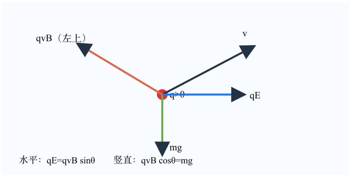
Figure 2: 受力分解图
