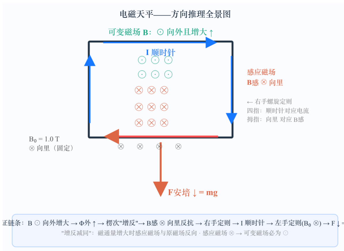
Figure 2: 电流方向与安培力
