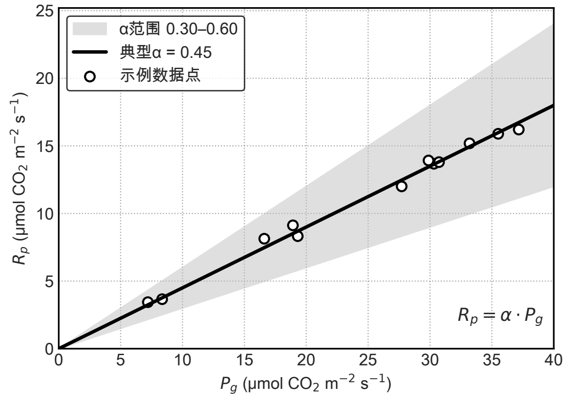
作物呼吸速率与总光合速率的线性关系
