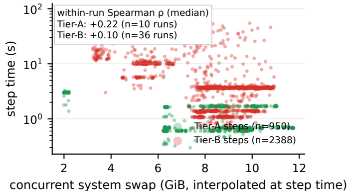
(d) step time vs concurrent swap (46 aligned runs)
