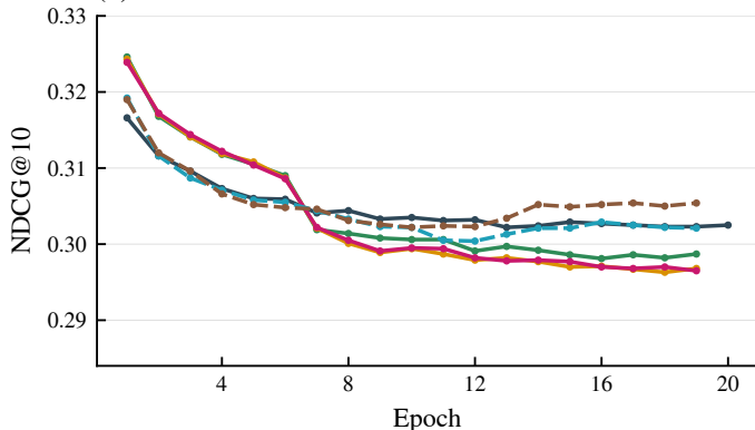
(d) ANCE · MS MARCO
