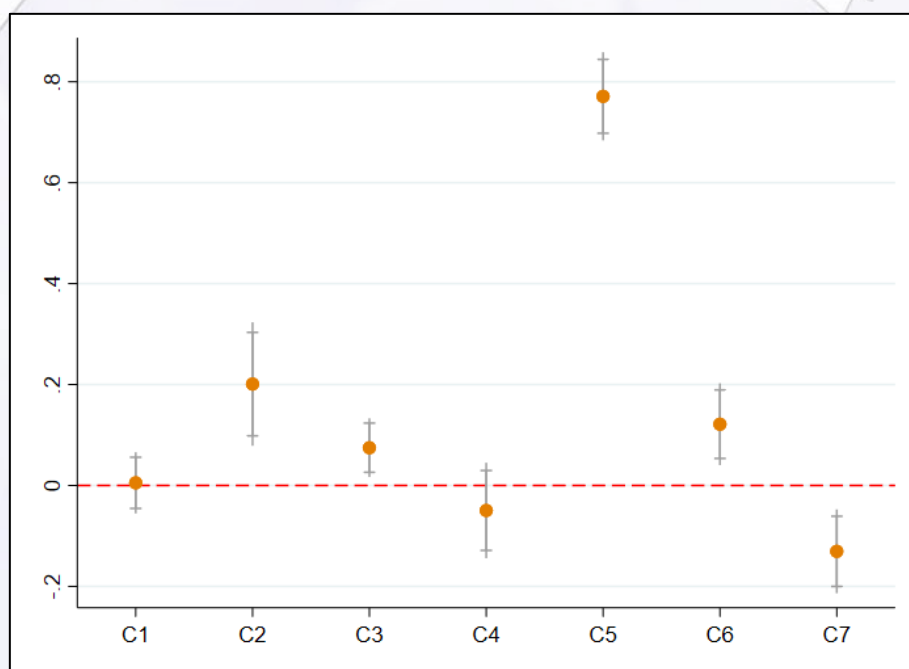
图21：回归系数可视化
