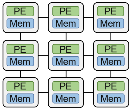
PE Array
