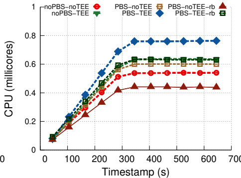
CPU: 210 TPS
