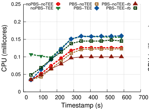
CPU: 30 TPS
