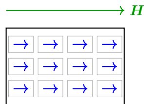
(b) 磁化饱和 外场对齐磁畴 \langle \mathbf{M} \rangle \neq 0
