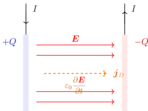
电容器极板间：位移电流接上传导电流的断裂
