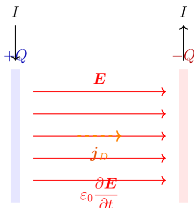
电容器极板间：位移电流接上传导电流的断裂
