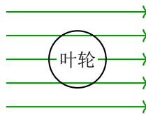
(b) 无旋场 \nabla \times \mathbf{A} = 0 叶轮不转
