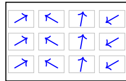
(a) 未磁化 磁畴随机取向 \langle \mathbf{M} \rangle = 0
